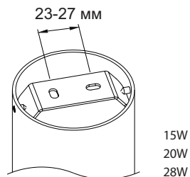
Рис.2. Схемf монтажа
