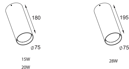
Рис.1. Габаритные размеры
