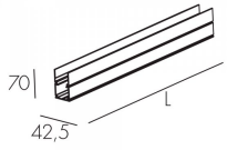
P18073321 Монтажный профиль Osio Pil 1257
